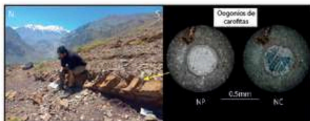
Figura 4. Imagen izquierda: Vista hacia el este de rocas de la Unidad Las Coloradas en el conón del Cerro Retumbadero, a la derecha: microfósiles llamados oógonos de carofitas, estos son el aparato reproductor de una planta subacuática (Charophyta).
