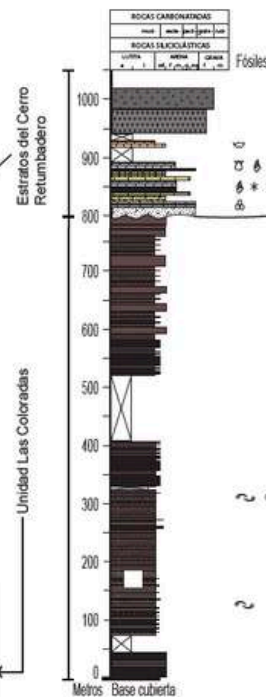
Figura 5. Sección estratigráfica realizada en la ladera del Cerro Las Américas.
