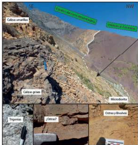
Figura 1. Imagen superior: vista hacia el suroeste en la ladera del conón del Cerro Retumbadero, mostrando las rocas estudiadas. Imágenes inferiores: fotografías de fósiles encontrados en rocas de los Estratos del Cerro Retumbadero.
