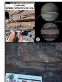
Figura 2. Estructuras sedimentarias observadas en rocas de la Unidad Las Coloradas A y C; en B se muestra una microfotografía tomada en un microscopio petrográfico.
